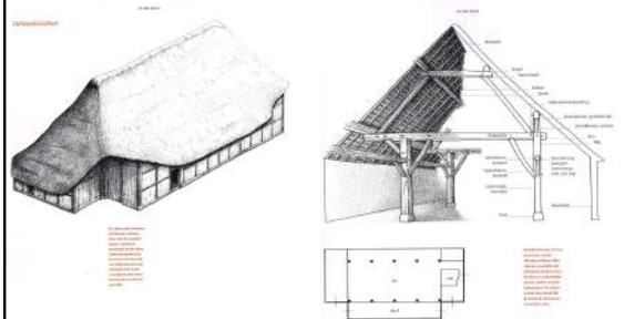
(zij) langsdeel (Vlaamse) schuur
