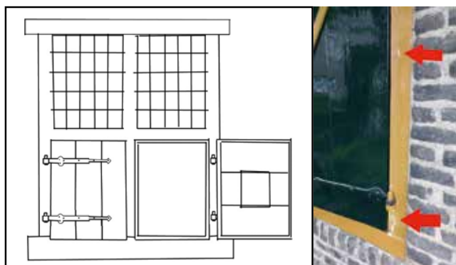
Links een tekening van een kruiskozijn met glas-in-lood in de bovenlichten en onderramen zonder glas, maar met (halfhoge) luiken. Rechts het onderste deel van een raamkozijn van De Blauwe Kei, waar de rode pijlen aangeven waar houten stoppen zijn aangebracht in de vroegere duimgaten. De onderste duim van het 'nieuwe' hoge luik zit ietsje hoger dan het oude duimgat.
